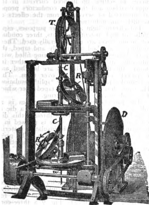
FIG. 2.—Taping Machine.
