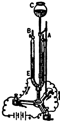
FIG. 2.—Water Voltmeter.
