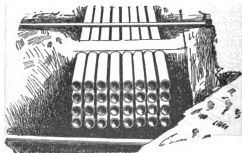
FIG. 13.—Cement-lined Conduit.
