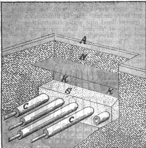
FIG. 10.—Sidewalk Conduit.
